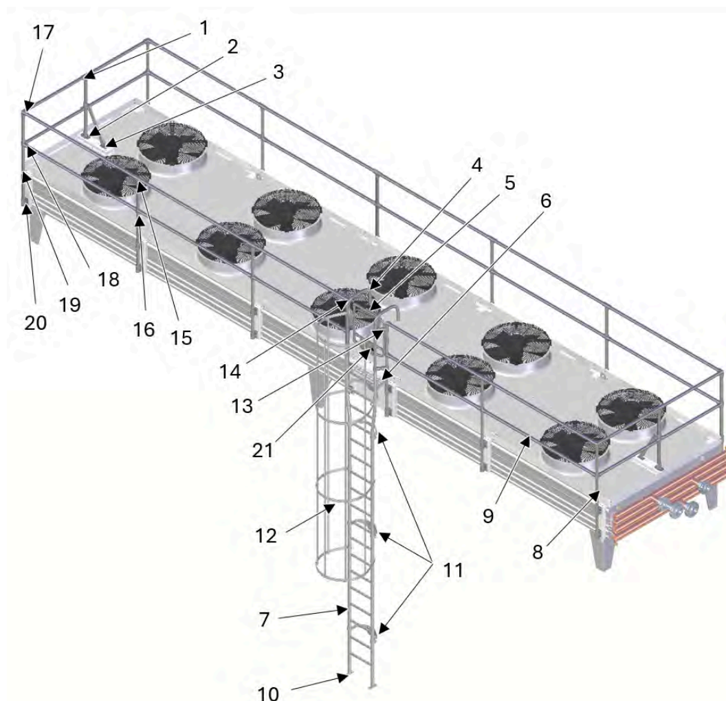
Einreihige Absturzsicherung
